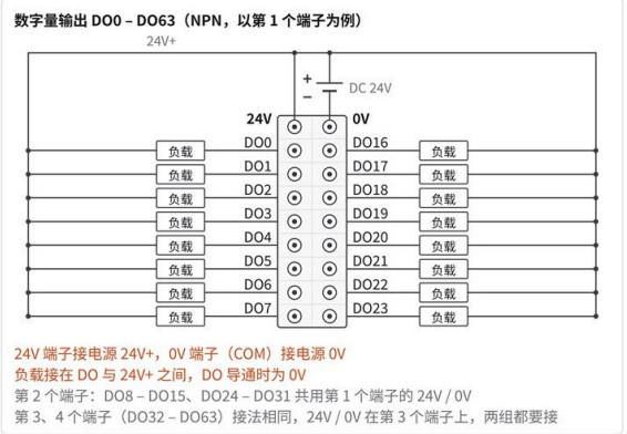
图 6-3 EP6464DN 接口与接线
