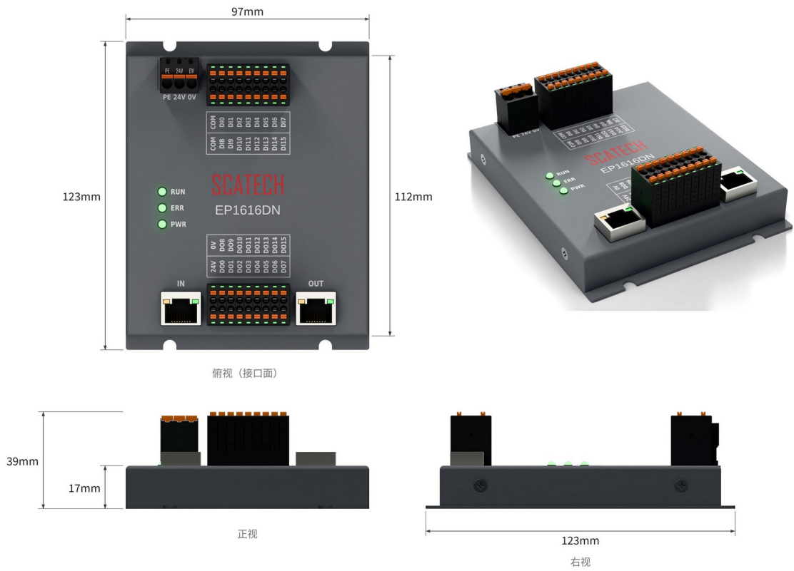
图 9-1 EP1616DN (单位: mm)
