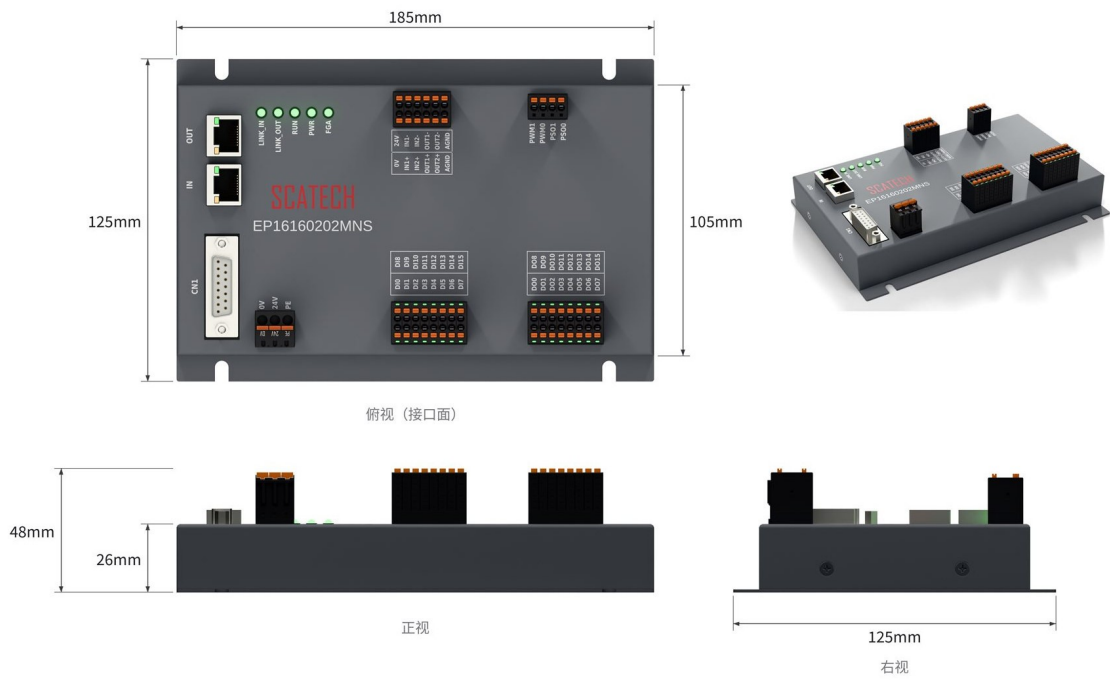
图 9-4 EP16160202MNS（单位：mm）
