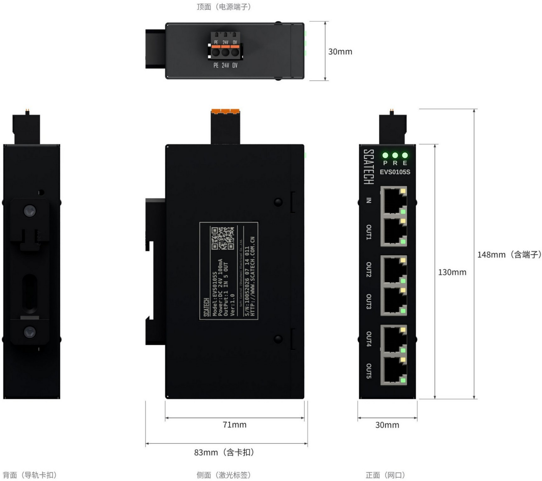
EVS0105S 外形尺寸（单位：mm）
